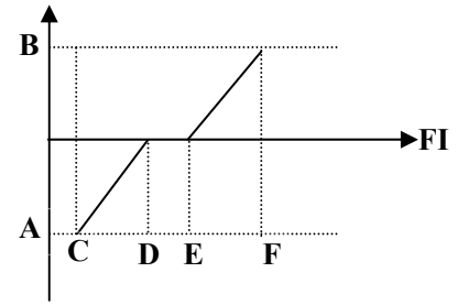
Рис 5-10 Комбинированный контроль
