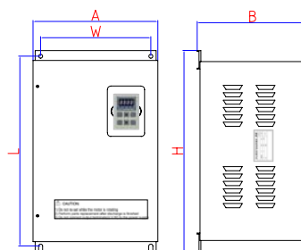
Металлический шкаф
